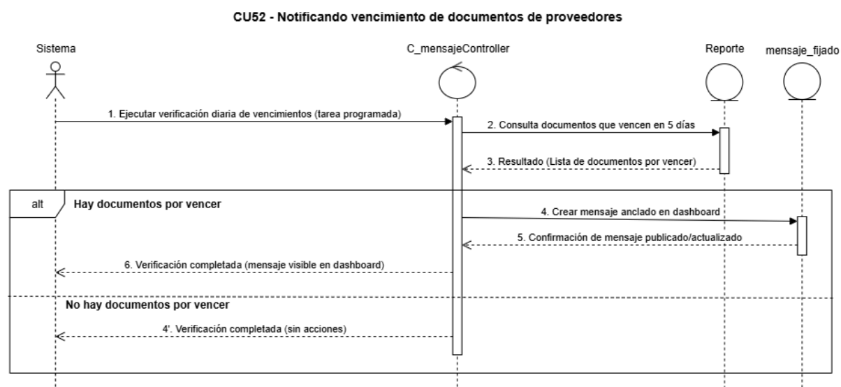
Figura 132, diagrama de secuencia CU N°52
