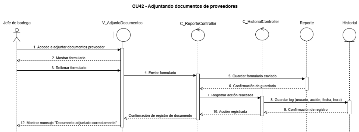
Figura 97, diagrama de secuencia CU N°42
