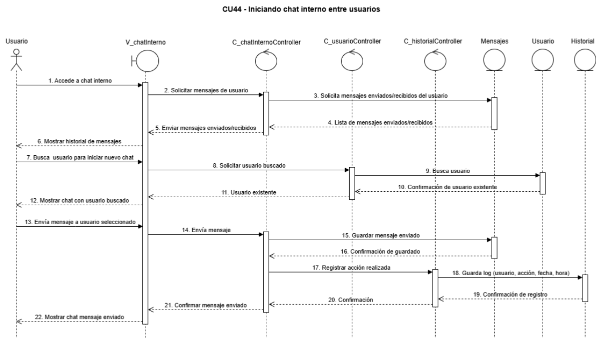
Figura 105, diagrama de secuencia CU N°44
