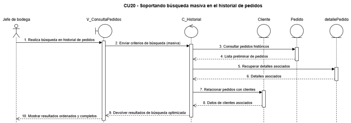
Figura 29, diagrama de secuencia CU N°20
