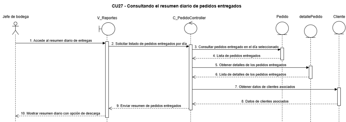
Figura 52, diagrama de secuencia CU N°27
