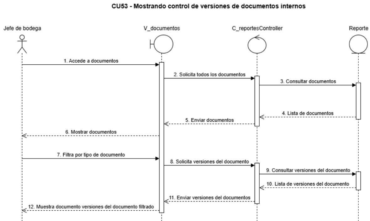
Figura 135, diagrama de secuencia CU N°53
