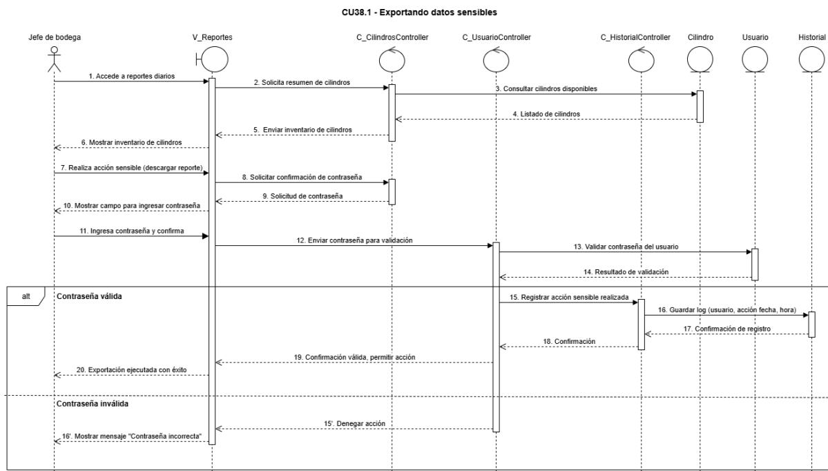
Figura 84, diagrama de secuencia CU N°38.1
