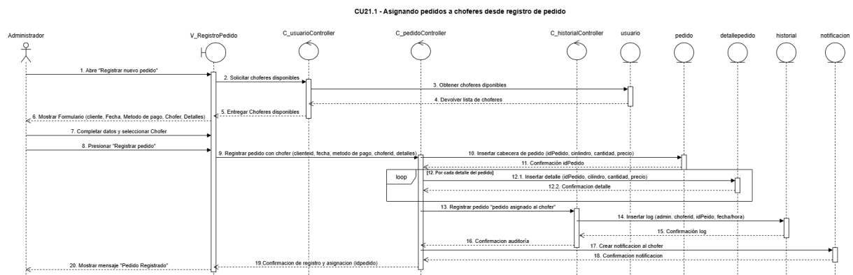
Figura 32, diagrama de secuencia CU N°21.1
