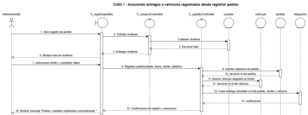
Figura 151, diagrama de secuencia CU N°63.1
