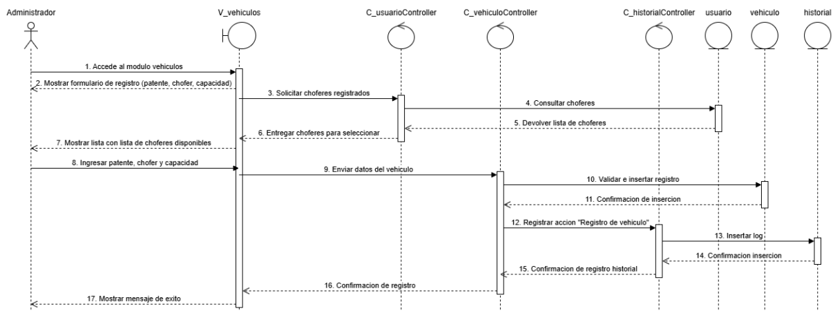
Figura 109, diagrama de secuencia CU N°46
