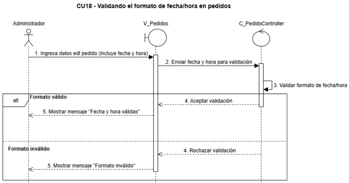
Figura 23, diagrama de secuencia CU N°18
