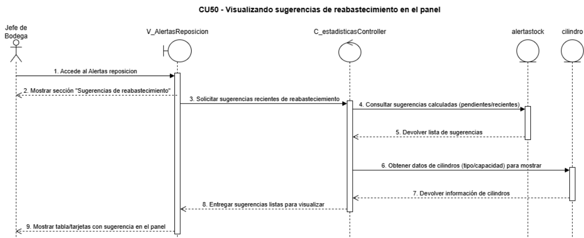
Figura 126, diagrama de secuencia CU N°50
