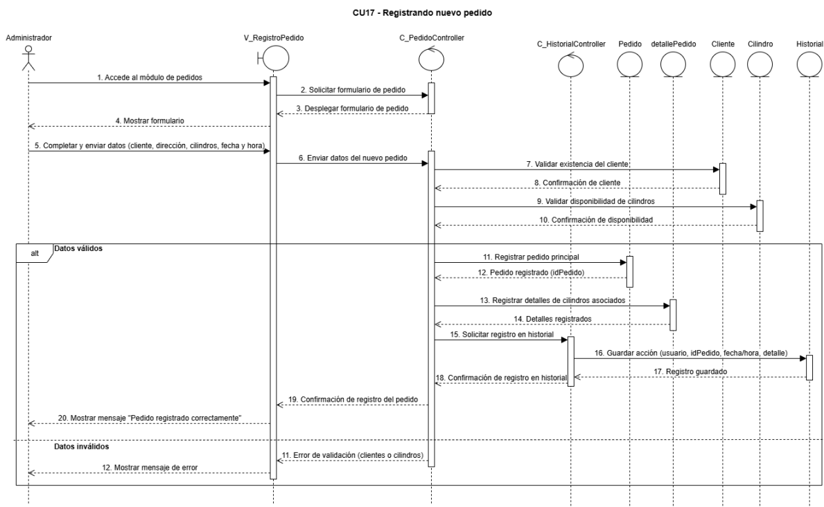
Figura 17, diagrama de secuencia CU 17
