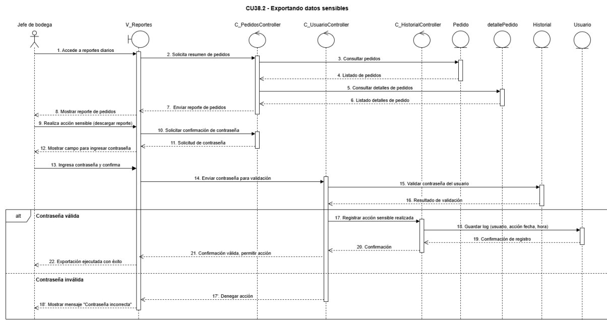
Figura 85, diagrama de secuencia CU N°38.2
