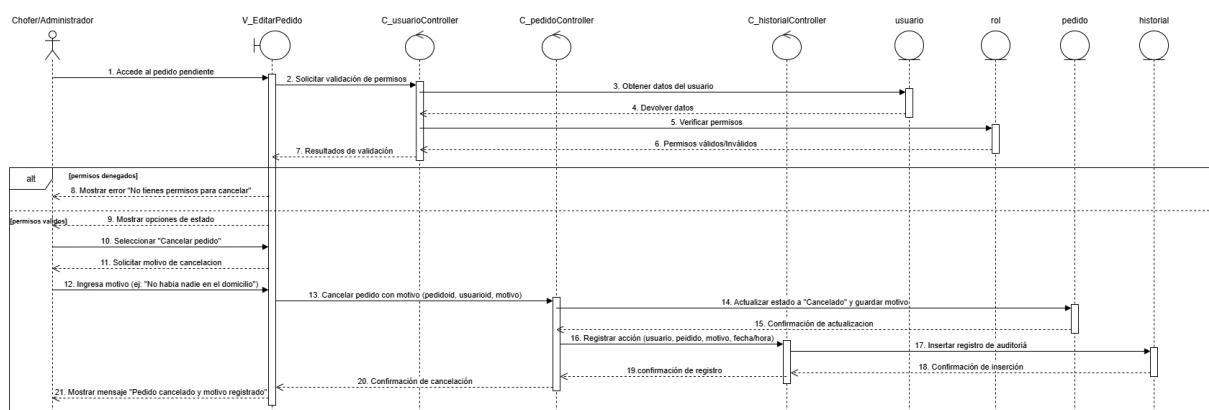
Figura 13, diagrama de secuencia CU N°16.
