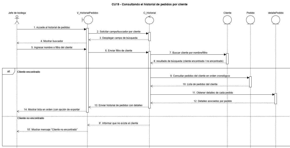
Figura 26, diagrama de secuencia CU N°19
