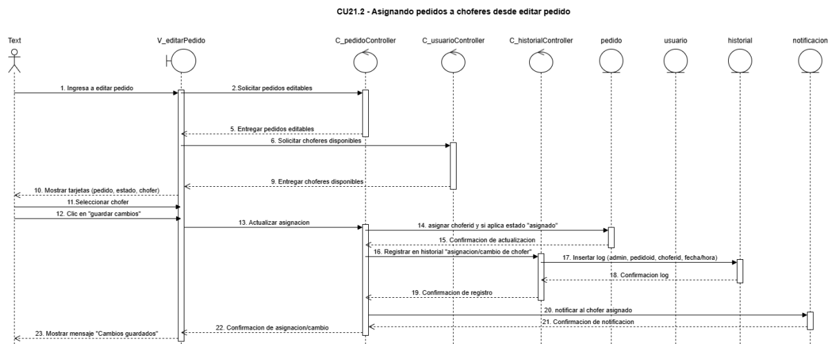
Figura 33, diagrama de secuencia CU N° 21.2
