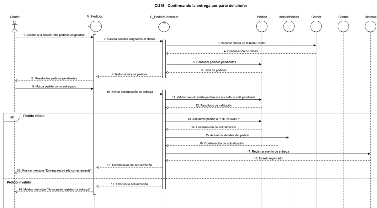
Figura 8, diagrama de secuencia CU N°15.
