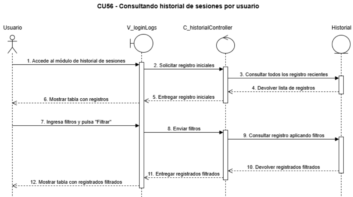
Figura 141, diagrama de secuencia CU N°56
