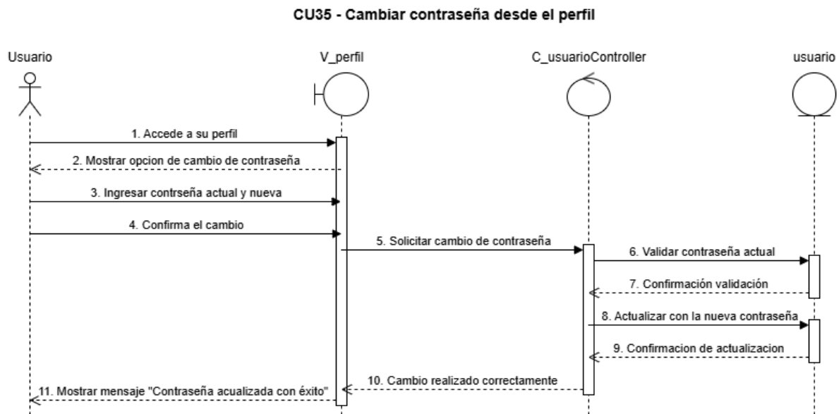
Figura 77, diagrama de secuencia CU N°35
