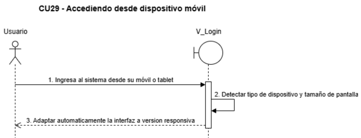
Figura 59, diagrama de secuencia CU N°29.
