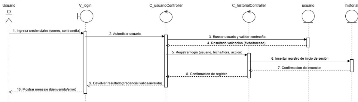
Figura 93, diagrama de secuencia CU N°41
