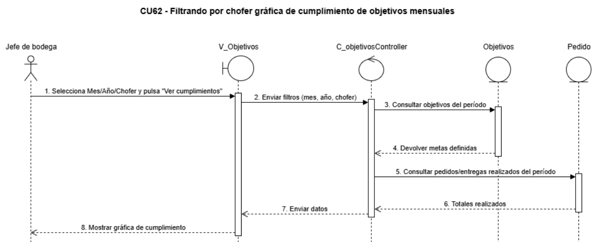
Figura 148, diagrama de secuencia CU N°62
