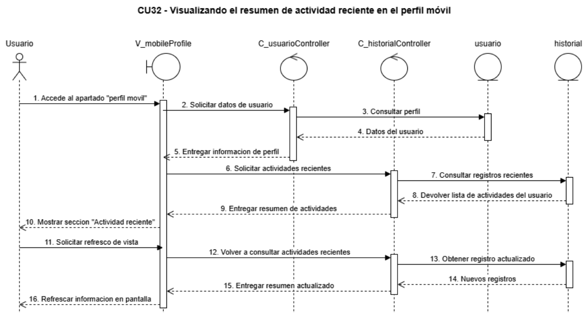
Figura 66, diagrama de secuencia CU N°32
