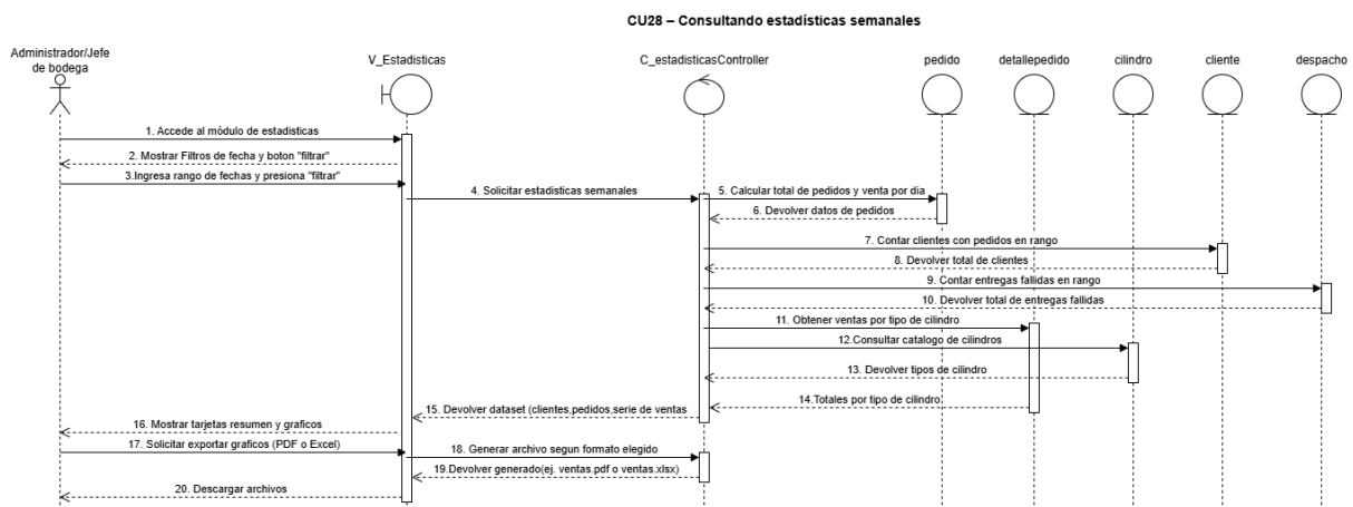
Figura 55, diagrama de secuencia CU N°28
