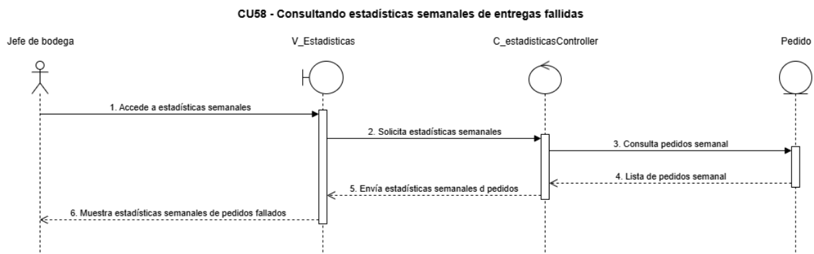
Figura 145, diagrama de secuencia CU N°58
