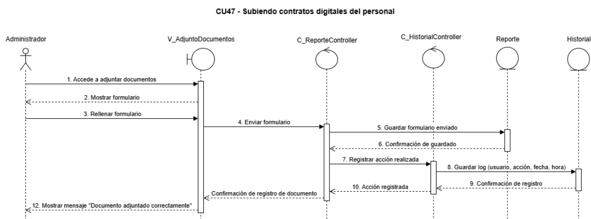
Figura 114, diagrama de secuencia CU N°47
