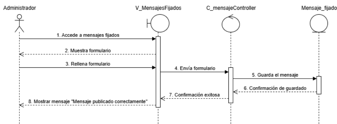
Figura 90, diagrama de secuencia CU N°39
