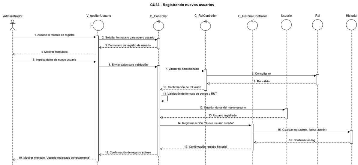
Figura 69, diagrama de secuencia CU N°33
