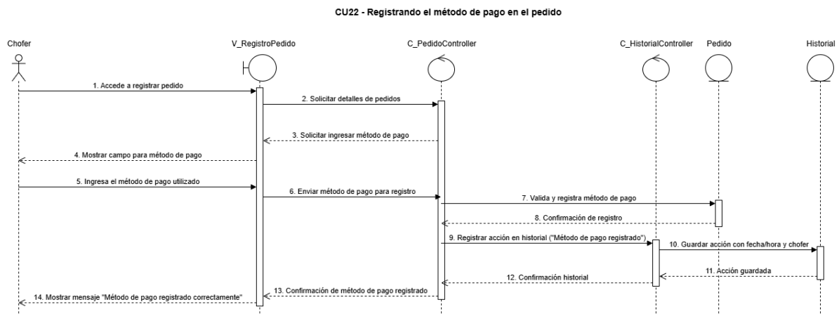
Figura 41, diagrama de secuencia CU N°22
