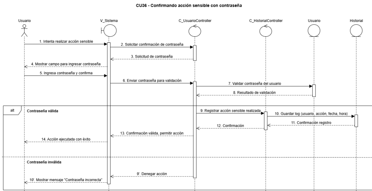
Figura 81, diagrama de secuencia
