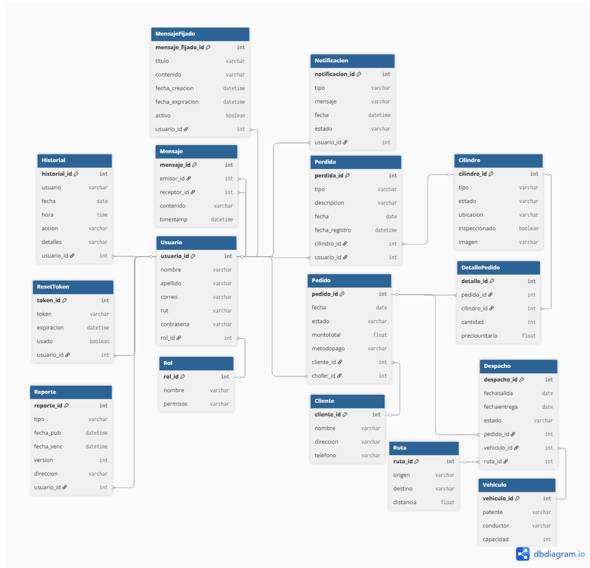
Figura 4. Diagrama de base de datos
