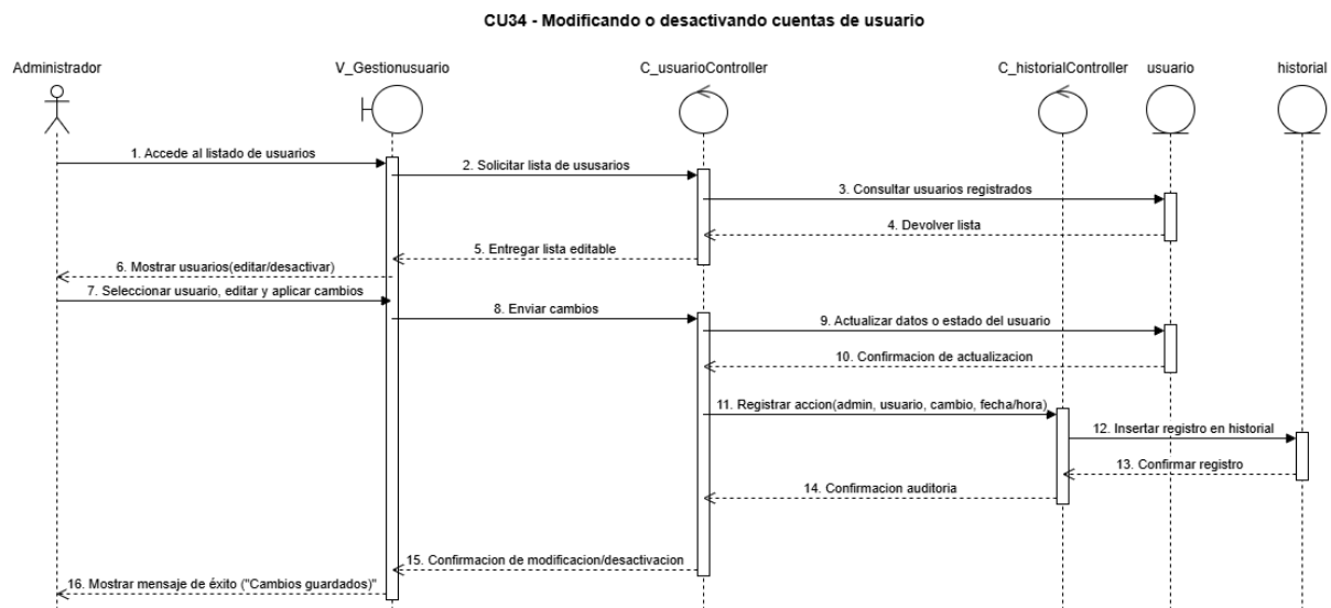
Figura 73, diagrama de secuencia CU N°34
