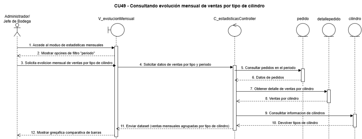
Figura 122, diagrama de secuencia CU N°49
