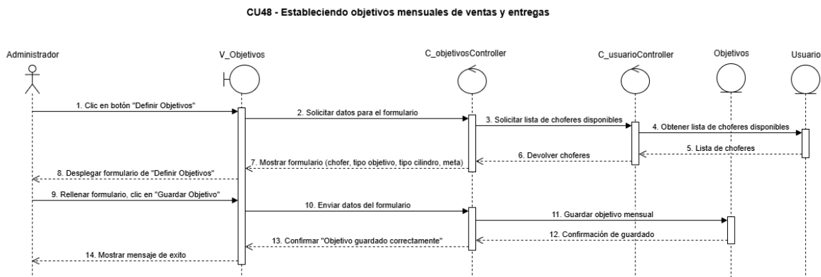
Figura 118, diagrama de secuencia CU N°48
