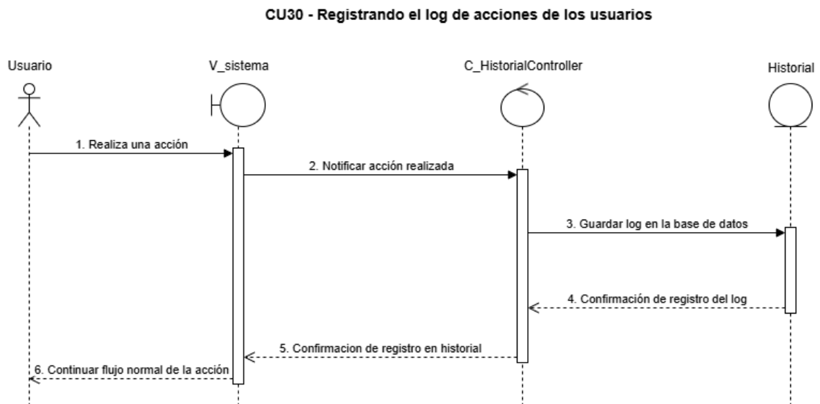
Figura 63, diagrama de secuencia CU N°30
