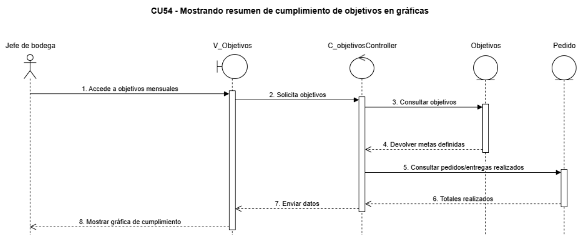
Figura 138, diagrama de secuencia CU N°54
