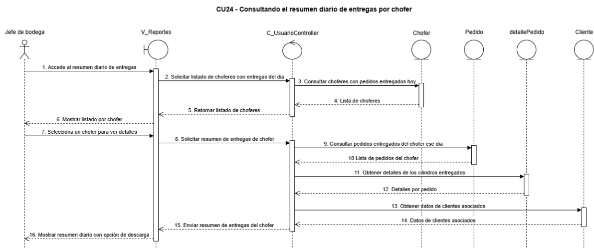
Figura 49, diagrama de secuencia CU N°24
