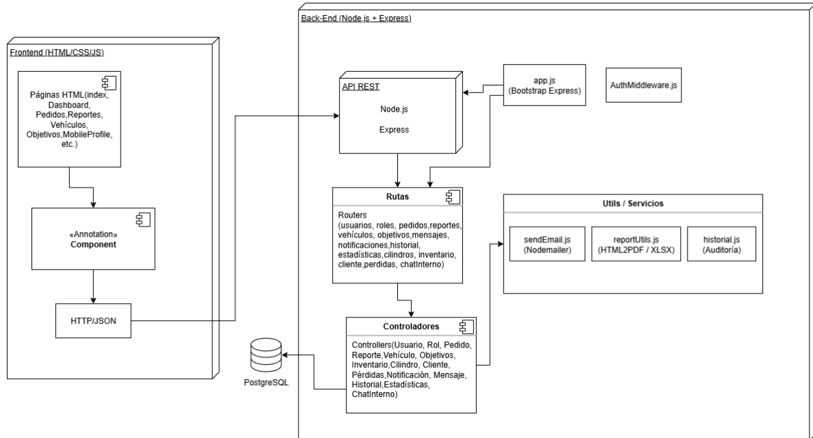
Figura 5, Diagrama de componentes
