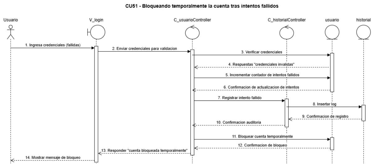
Figura 129, diagrama de secuencia CU N°51
