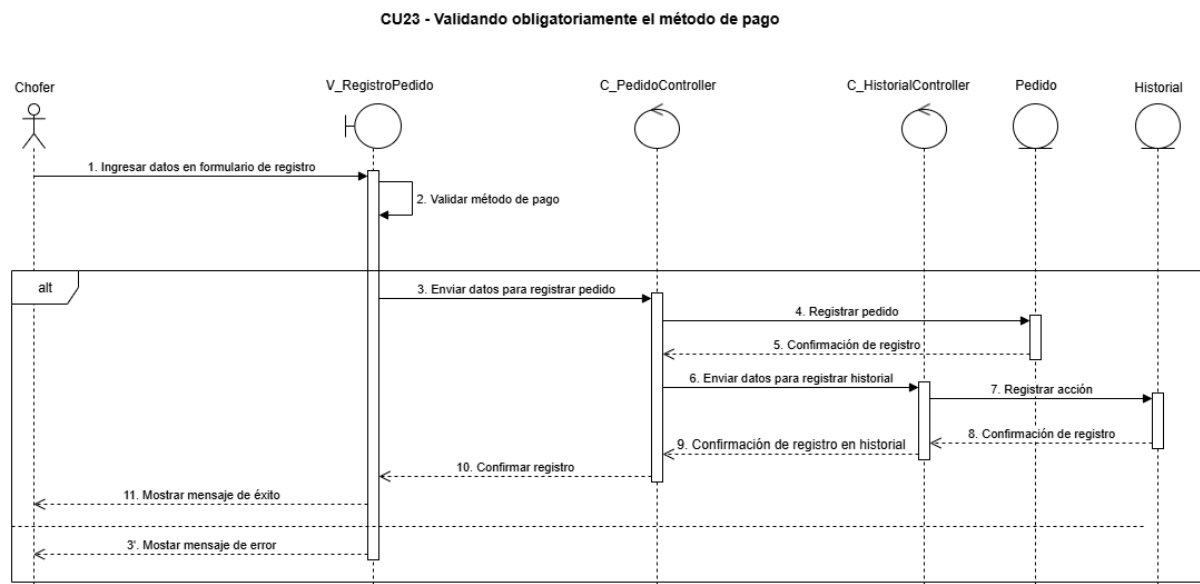
Figura 46, diagrama de secuencia CU N°23
